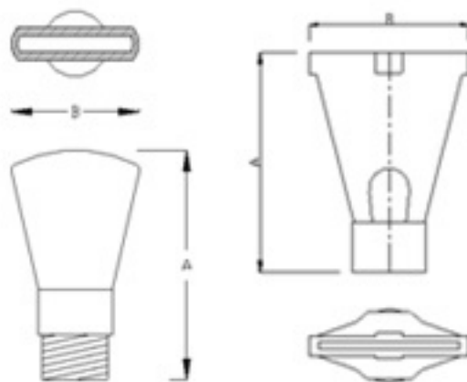
Rys. Dysza Fan-Jet w zespole z dyszą centralną
